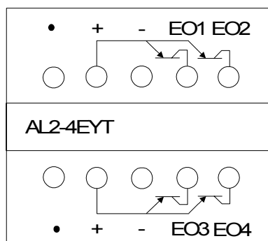
Illustrazione 5.10: AL2-4EYT, Uscita transistore
