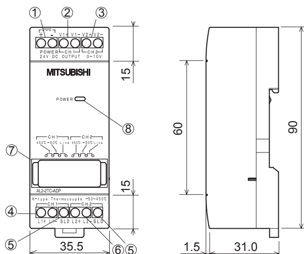
Figura 13.1: Dimensiones exteriores
