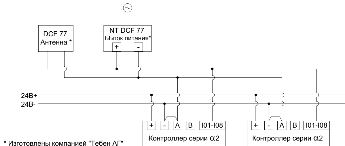
Рисунок 10.2: Электрические соединения
