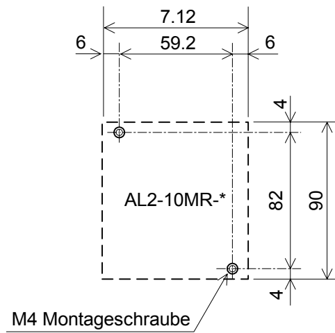
Abbildung 3.4: Direktmontage
