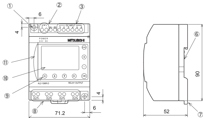
Abbildung 1.1: Bedienungselemente(AL2-10MR-*)
