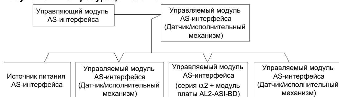
Рисунок 9.2: Конфигурация системы
