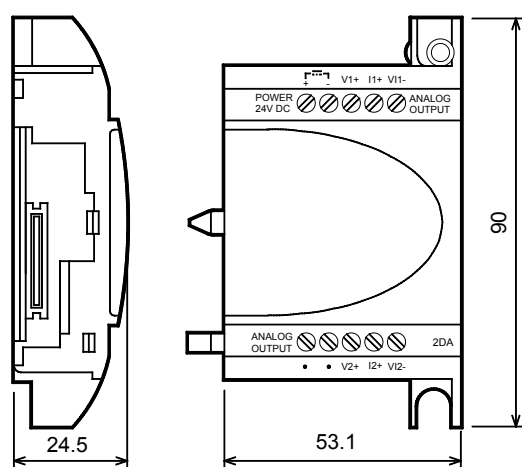
Figure 11.2: Dimensions extérieures
