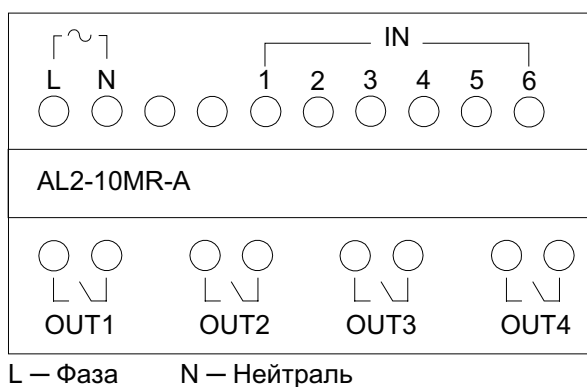
Рисунок 5.1: Устройство AL2-10MR-A, входные клеммы для подачи напряжений перемен. тока, выходные клеммы реле
