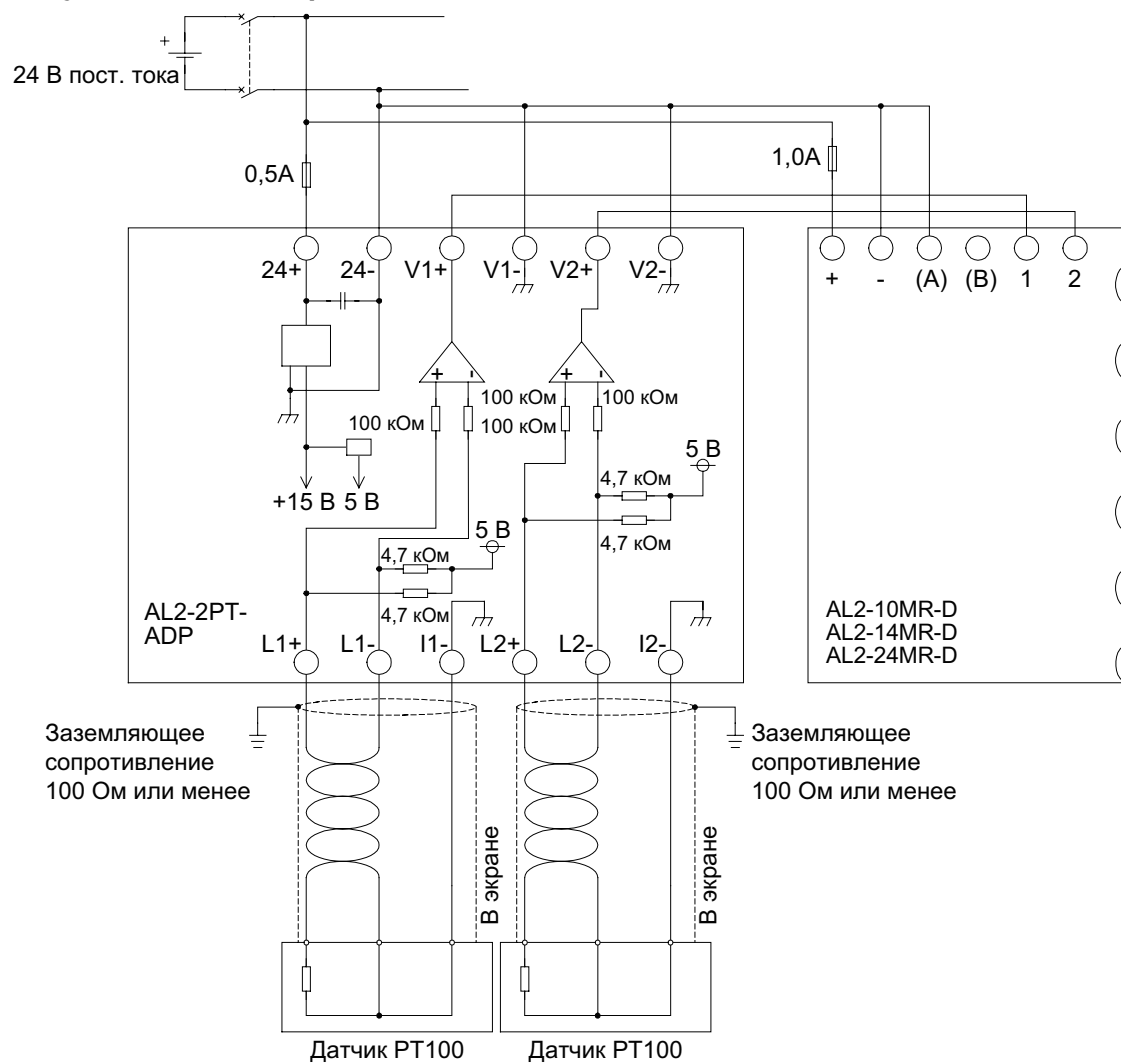
Рисунок 12.4: Электрические соединения
