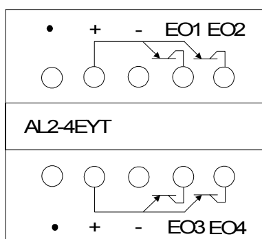
Figur 5.10: AL2-4EYT, transistorutgång
