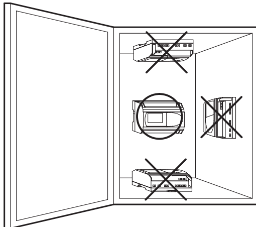
Abbildung 3.1: Montageanordnung
