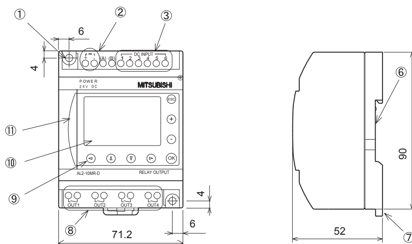
Figur 1.1: Benämningar(AL2-10MR-*)
