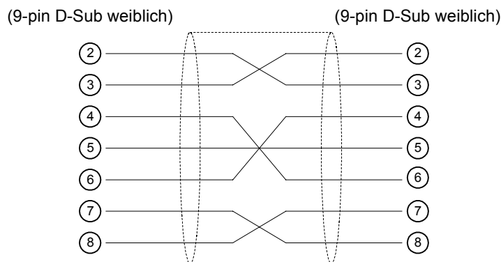
Abbildung 8.3: RS-232C serielltes Kabel Pin-Belegung
