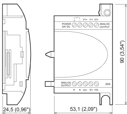
Рисунок 11.2: Внешние размеры
