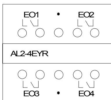
Illustrazione 5.9: AL2-4EYR, Uscita relè
