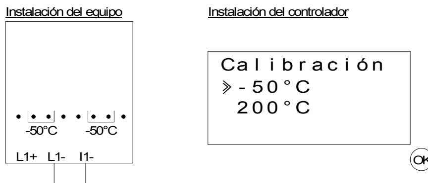
Figura 12.5: Compensación de la desviación en el AL2-2PT-ADP
