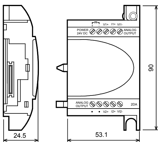
Figura 11.2: Dimensiones exteriores
