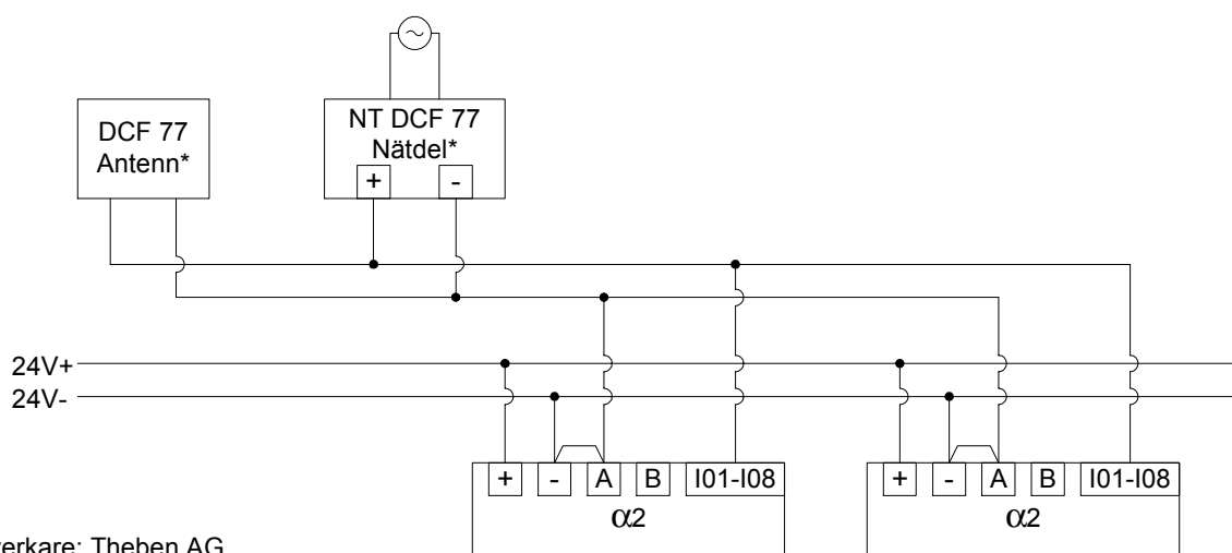
Figur 10.2: Anslutning av DCF77-antenn och nätrel
