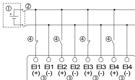
Figure 4.6: Plan de câblage de l'entrée source ("+" commun) AL2-4EX
