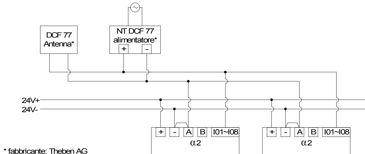
Illustrazione 10.2: Collegamento dell'antenna DCF77 e dell'alimentatore di rete
