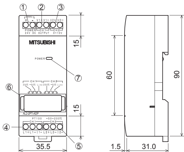
Figura 12.1: Dimensiones exteriores
