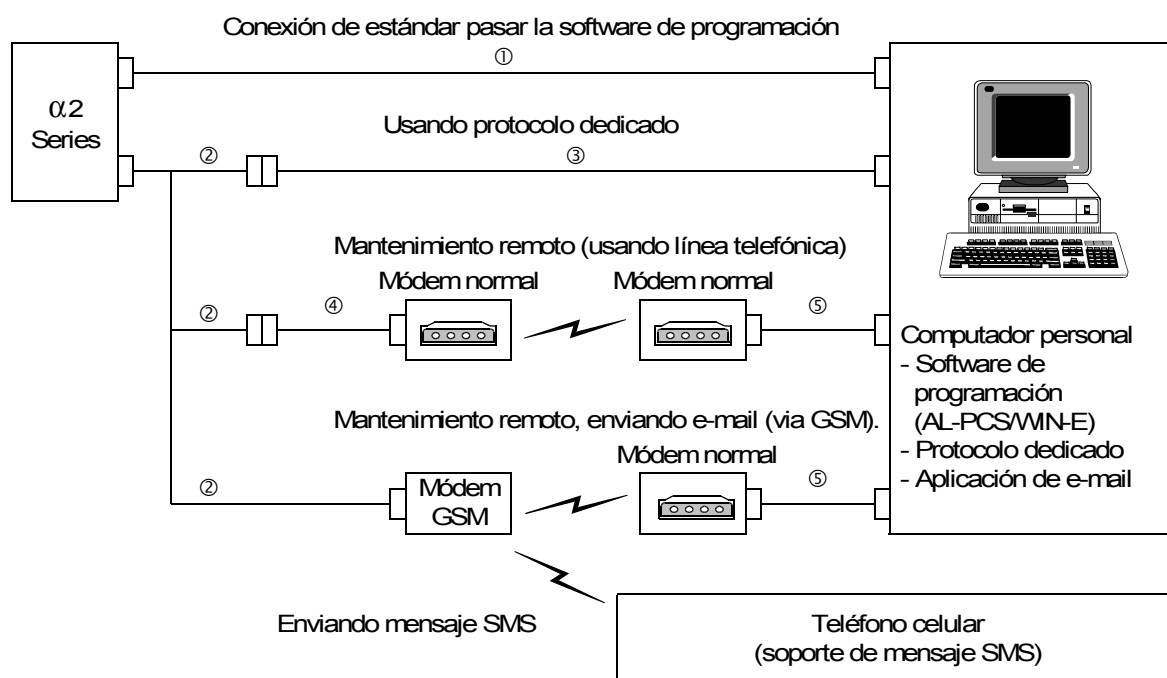
Figura 1.4: Configuración del sistema(AL2-14MR-*,AL2-24MR-*)
